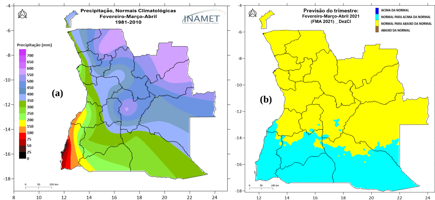
Figura 1: (a) Normais Climatológicas e (b) previsão do trimestre FMA 2021. Fonte: INAMET.
